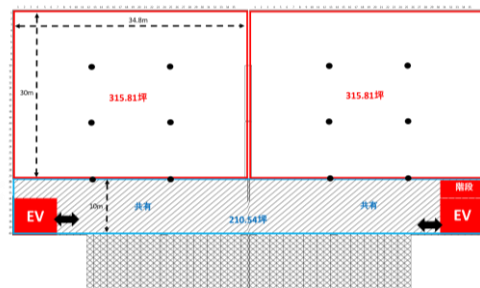
1階平面図
