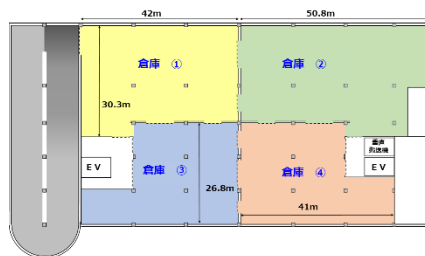
6階平面図
