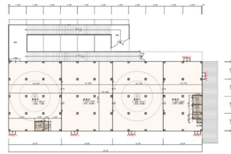
4階平面図
