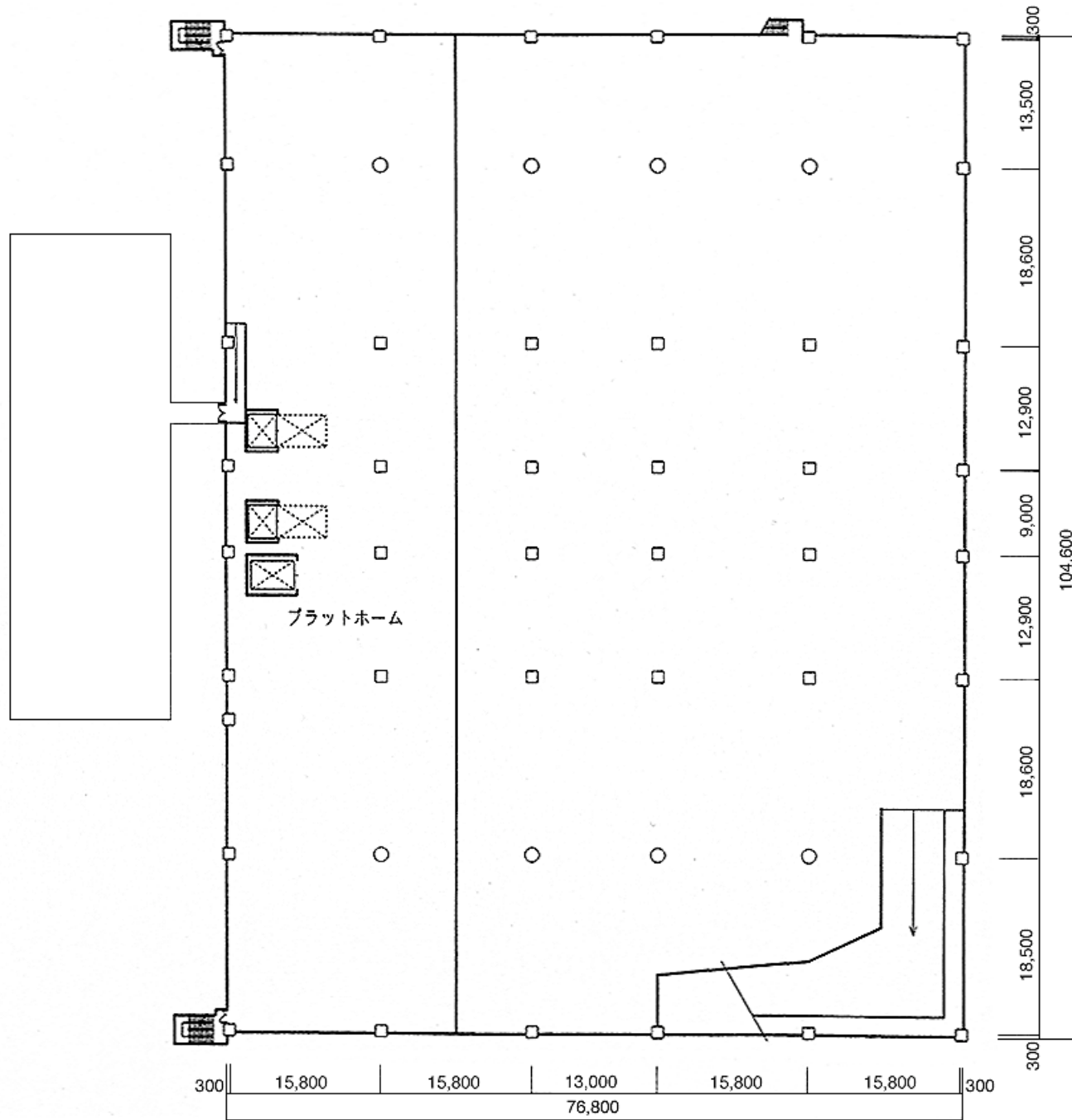
2F平面図
