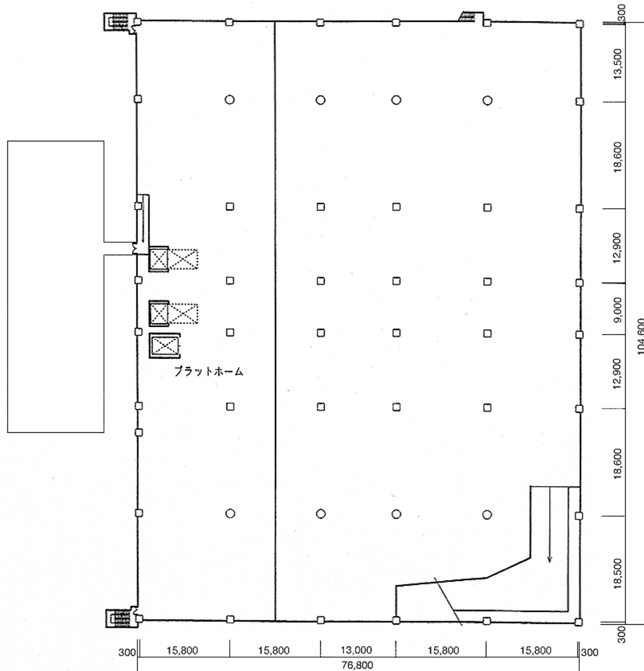
2F平面図
