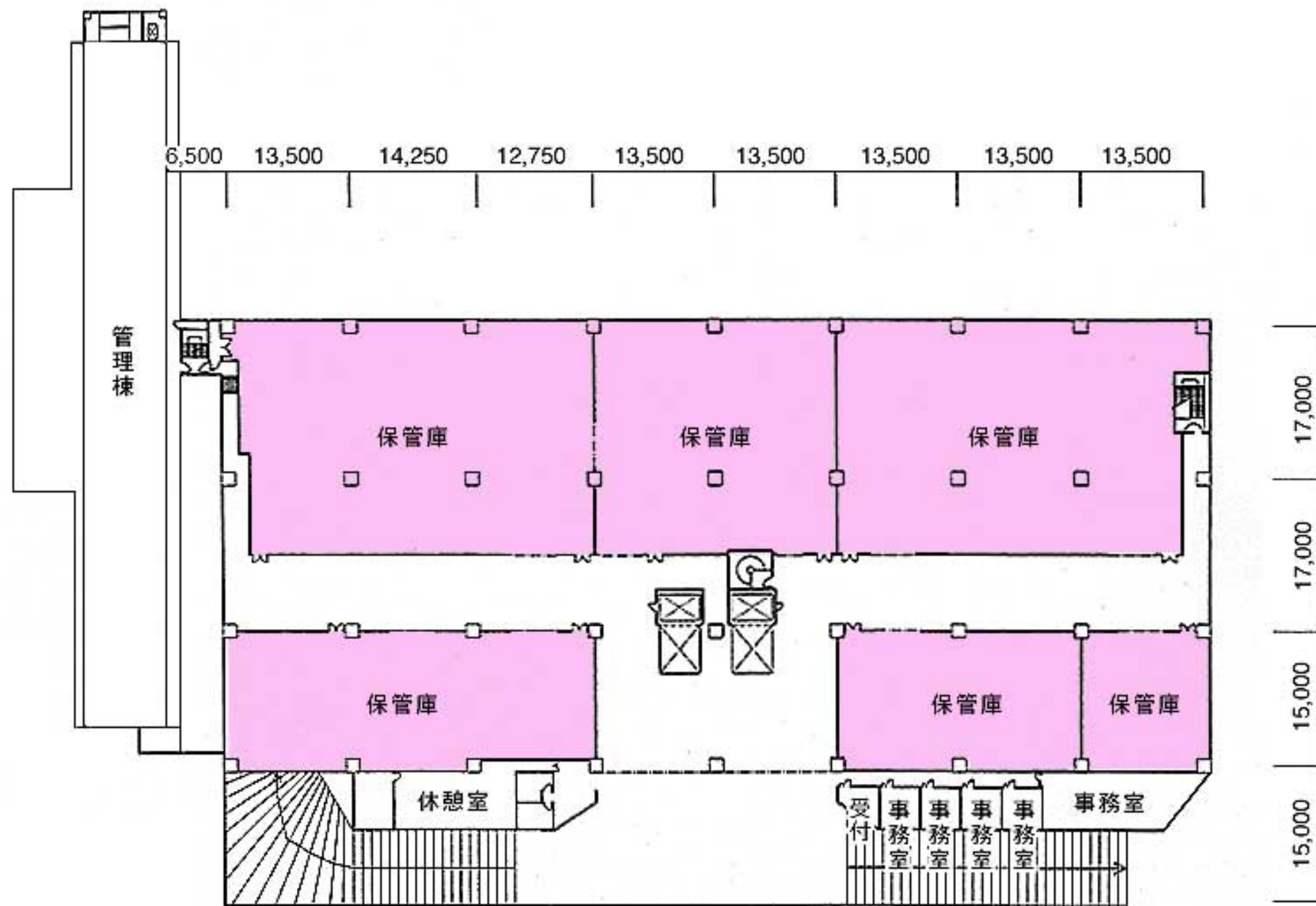
3F平面図
