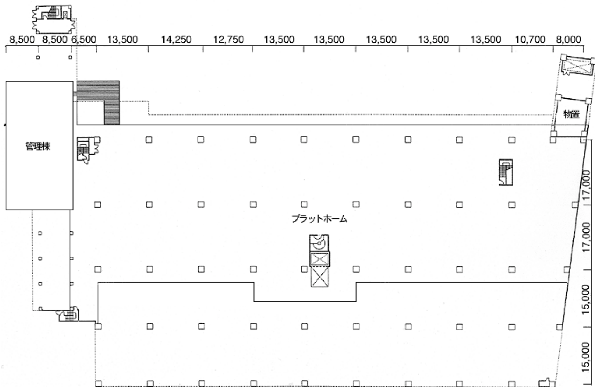
1F平面図
