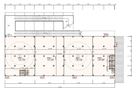
4階平面図
